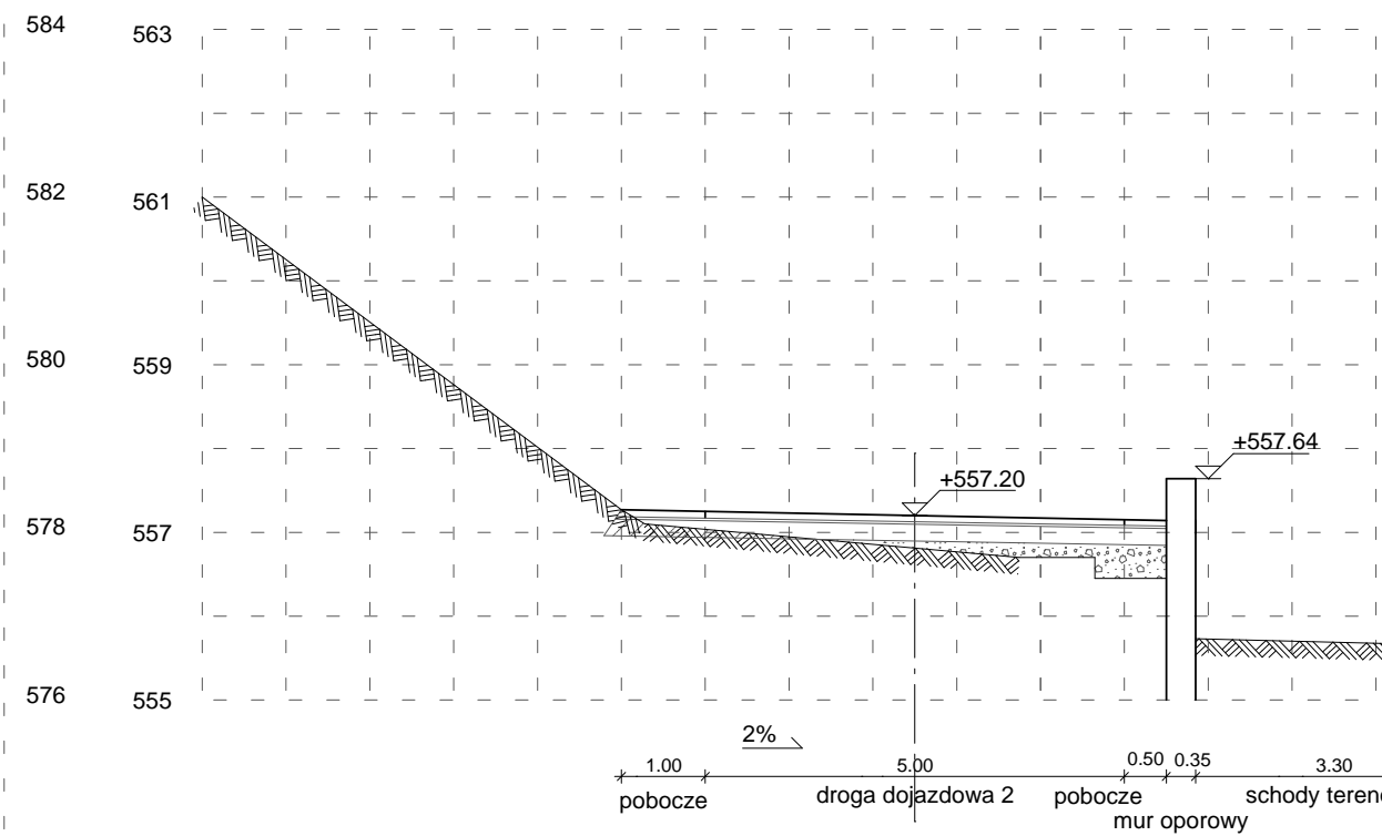
PRZEKRÓJ 06
