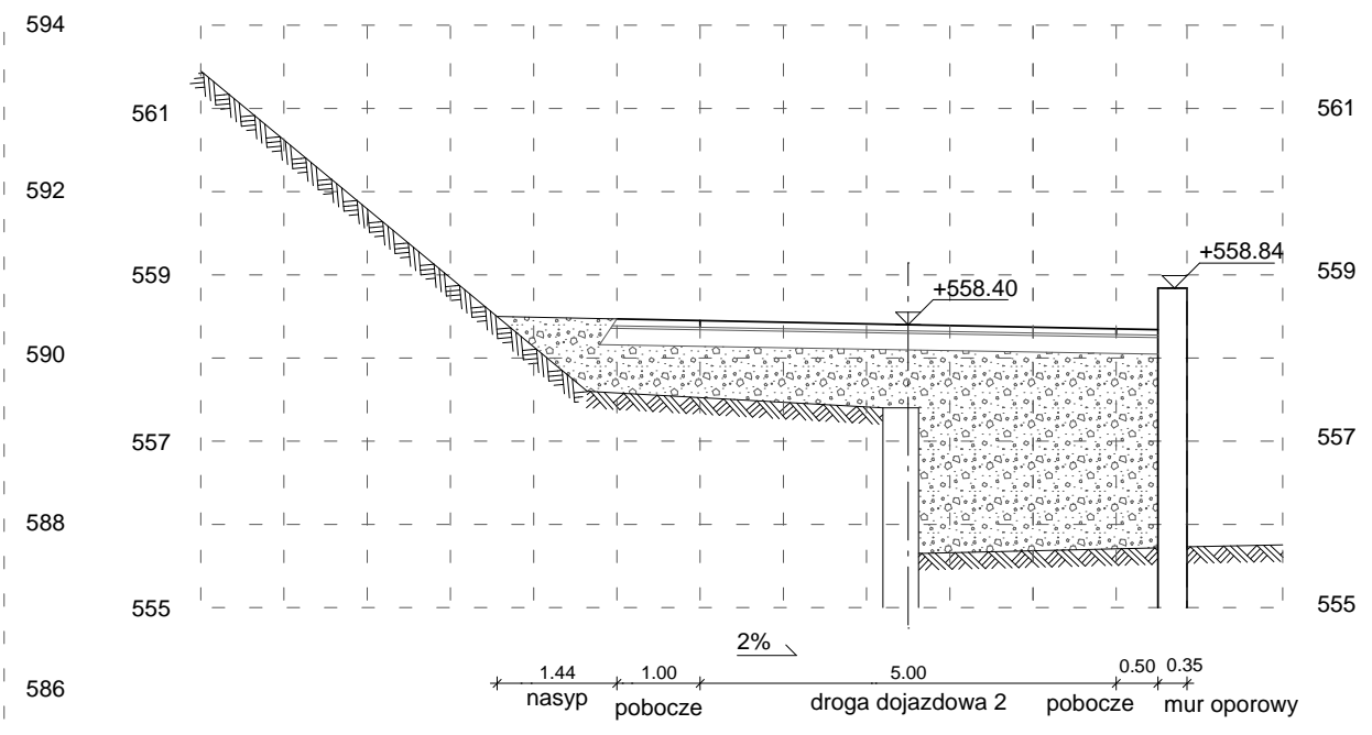
PRZEKRÓJ 06
