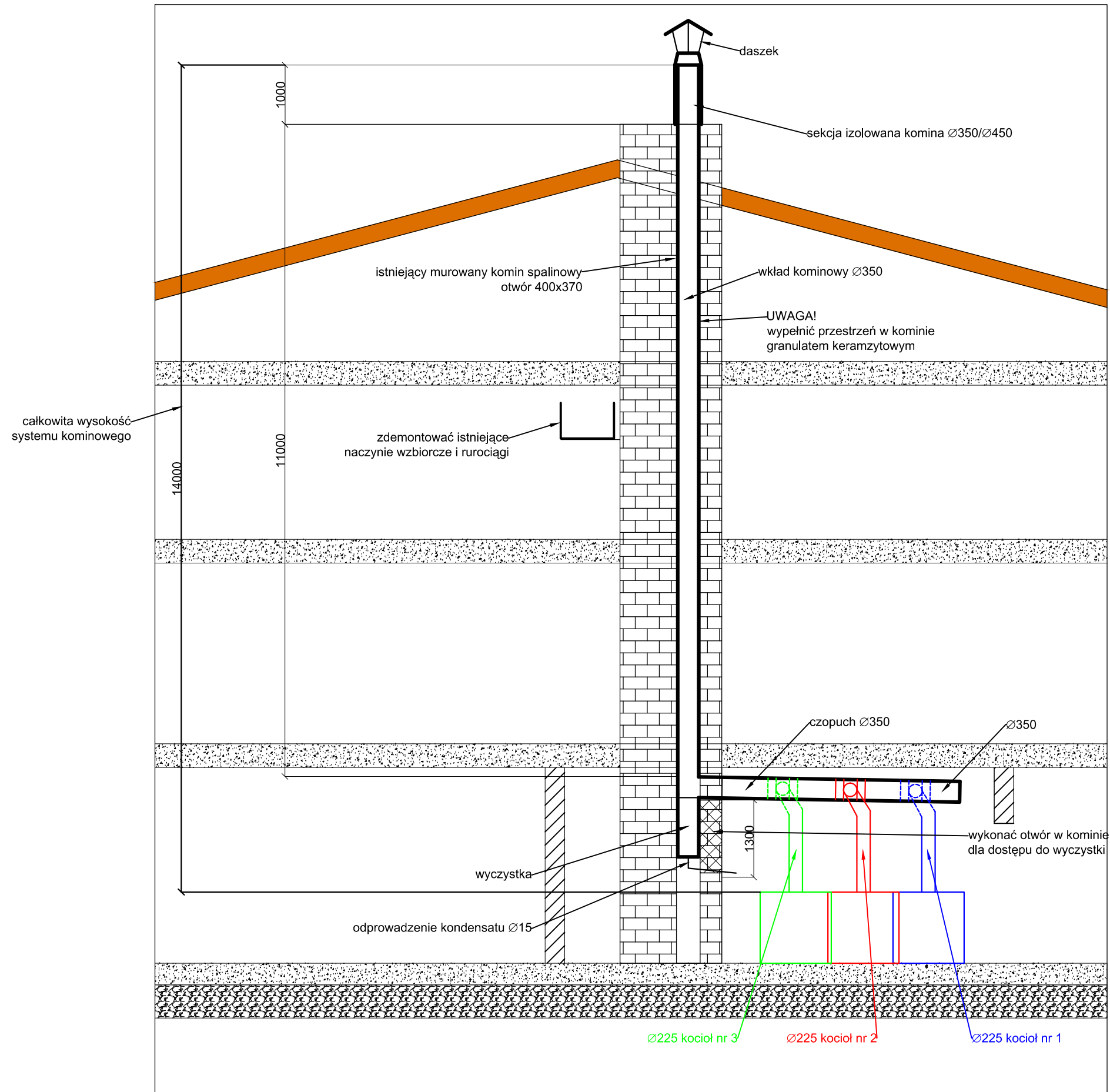
Przekrój komina spalinowego oraz sposób podłączenia kotłów
