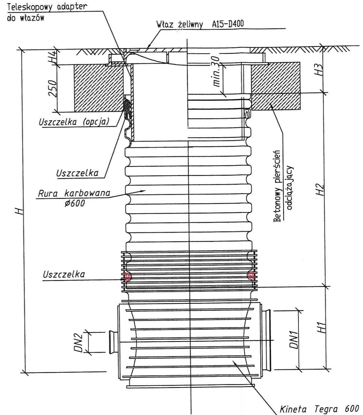
Studzienka rozprężna typu Tegra 600 z pierścieniem odciążającym
