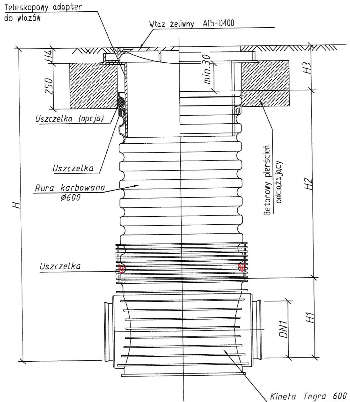
Studzienka inspekcyjna Tegra 600 z pierścieniem odciążającym
