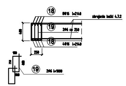
Poz. 4.7.5 25x40 szt. 1
