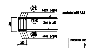
Poz. 4.7.7 25x40 szt. 1
