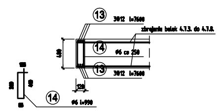
Poz. 4.7.2. 12x40 szt. 1
