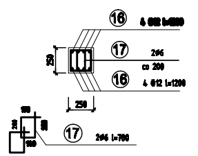
Poz. 4.7.4. 25x25 szt. 1
