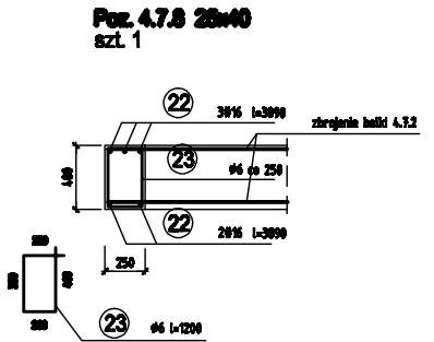
Zestawienie stali zbrojeniowej
