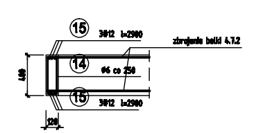
Poz. 4.7.3. 12x40 szt. 1
