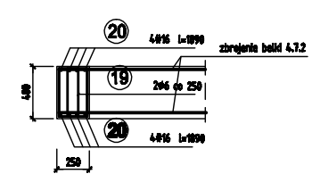
Poz. 4.7.6 25x40 szt. 1
