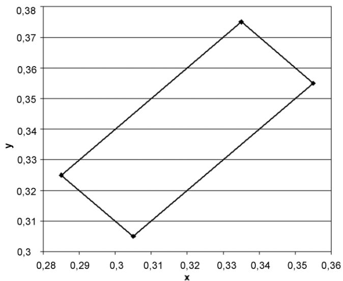
Rys. 1. Współrzędne chromatycyjnosc x,y dla barwy białej oznakowania
