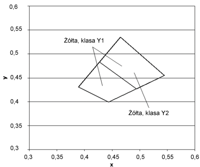
Rys.2. Współrzędne chromatycyjnosc x,y dla barwy żółtej oznakowania
